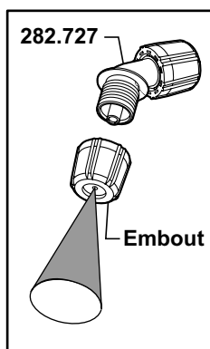
Buse complète
