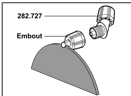
Buse complète
